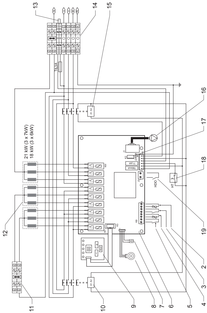
Электрическая схема котла ПРОТHERM Скот 21 (18) кВт
