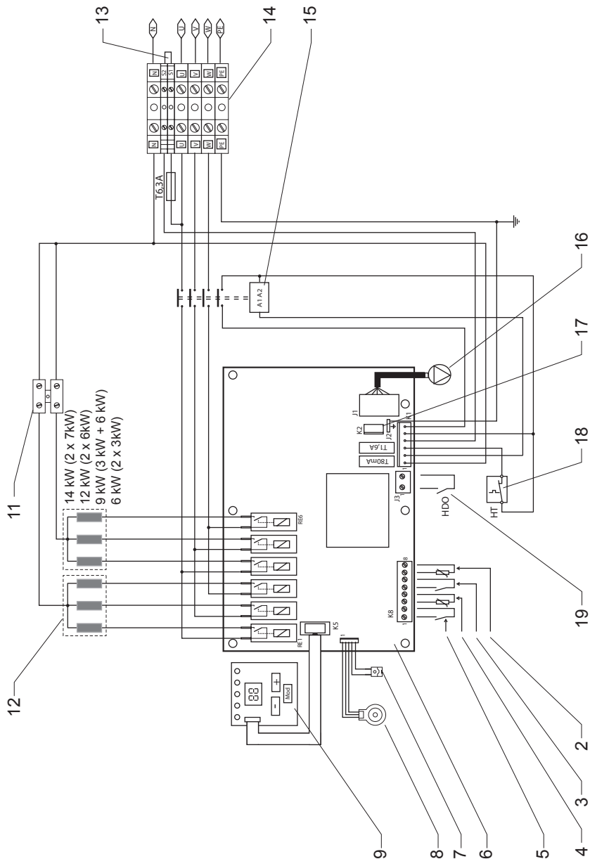
Электрическая схема котла ПРОТHERM Скот 14 (12, 9, 6) кВт
